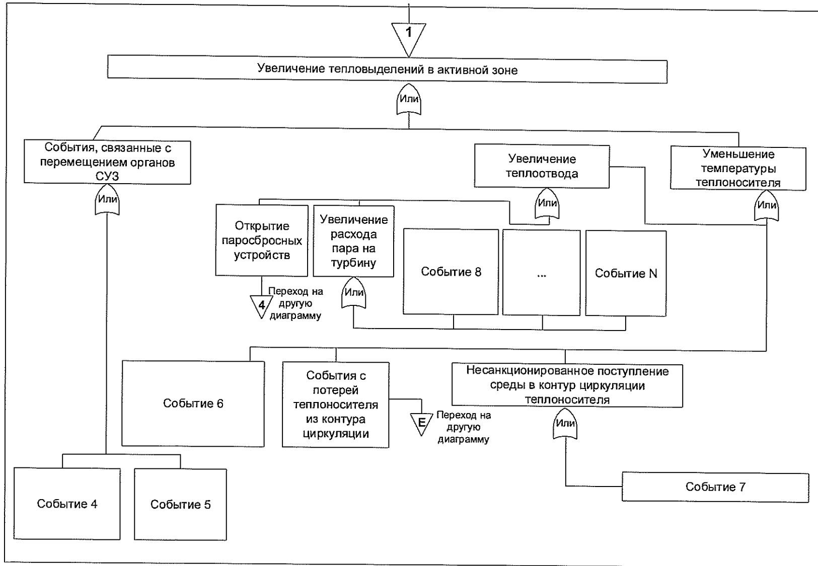
Рис. 2. Логическая диаграмма причин выхода РВ за установленные проектом границы (продолжение)
